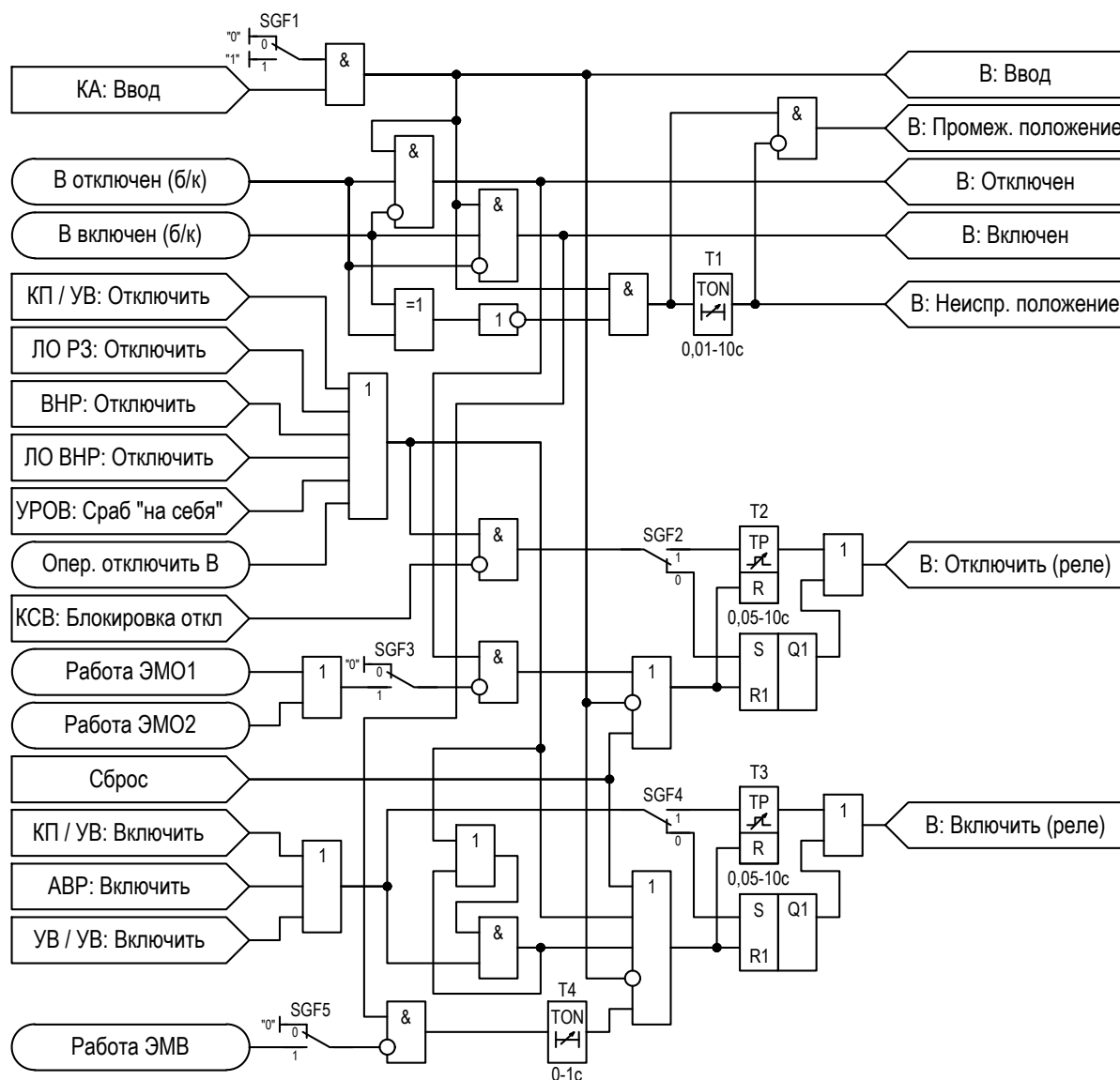
Рисунок 2.71 – Функциональная схема «Выключатель»
