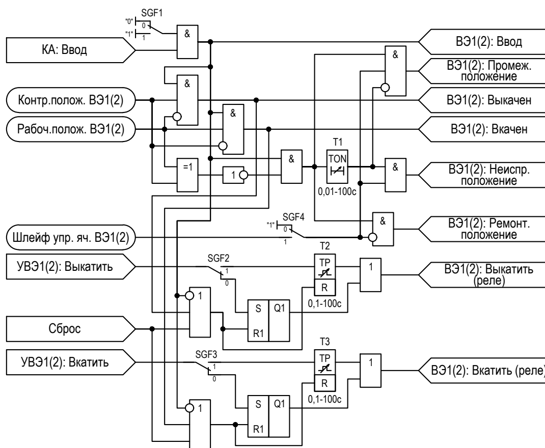
Рисунок 2.73 – Функциональная схема «ВЭ1(2)»
