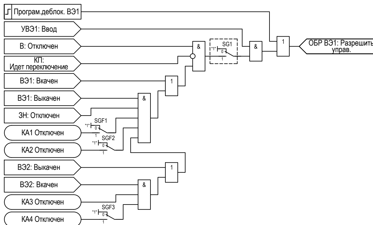
Рисунок 2.66 – Функциональная схема «ОБР ВЭ1»
