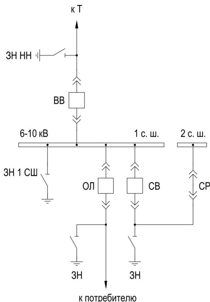
Рисунок 2.63 – Поясняющая схема первичной сети для алгоритмов оперативной блокировки КА
