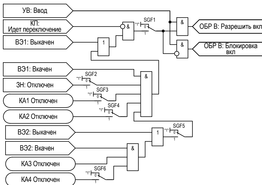
Рисунок 2.64 – Функциональная схема «ОБР В»
