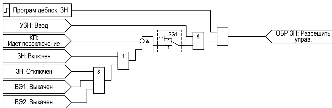
Рисунок 2.65 – Функциональная схема «ОБР ЗН»
