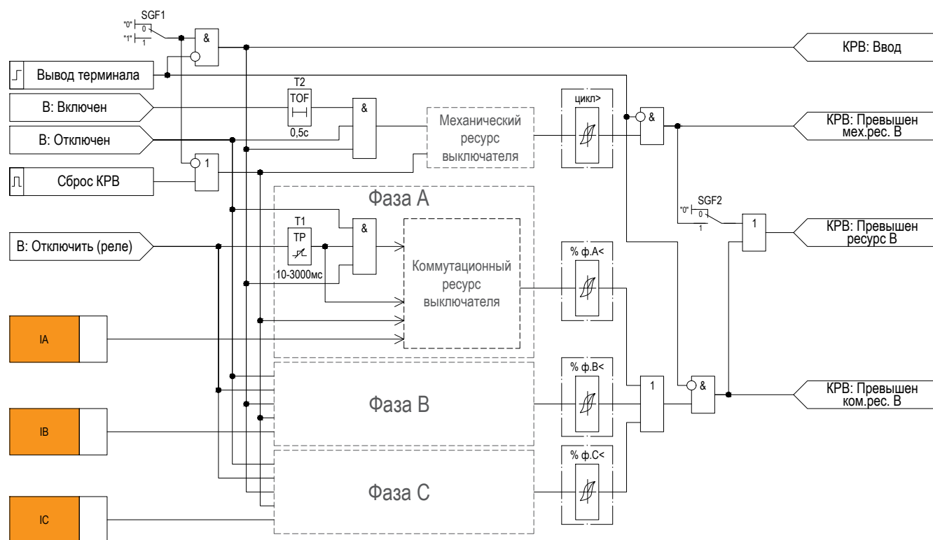
Рисунок 2.75 – Функциональная схема «КРВ»
