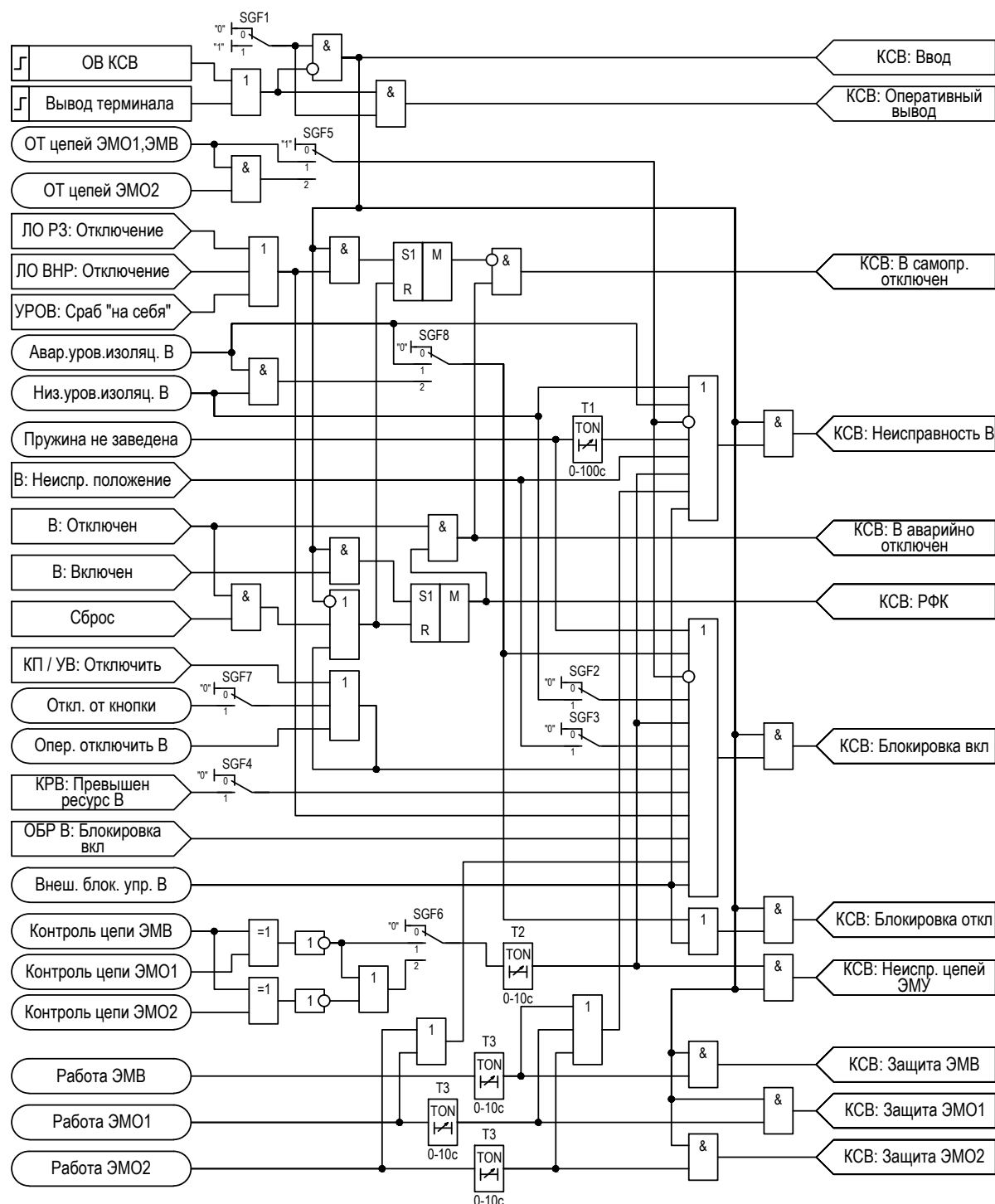
Рисунок 2.74 – Функциональная схема «КСВ»
