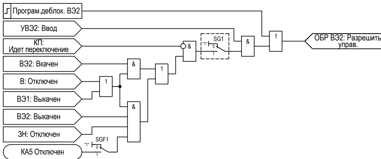
Рисунок 2.67 – Функциональная схема «ОБР ВЭ2»
