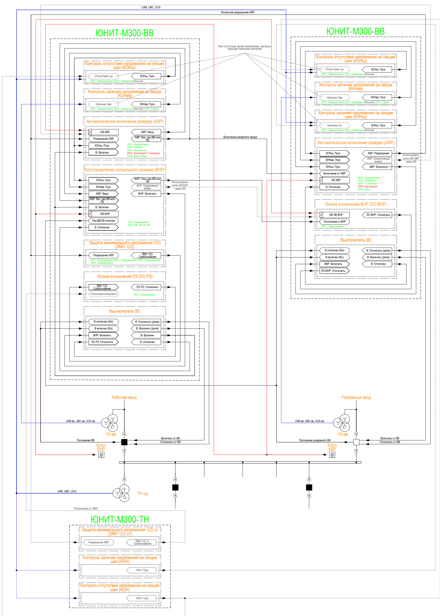
Рисунок К.2 – Поясняющая схема организации цепей ABP и BNR для первичной схемы с одним рабочим и одним секционным выключателями
