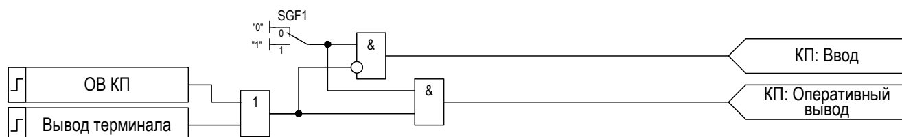
Рисунок 2.53 – Функциональная схема управления режимами работы функционального блока «КП»
