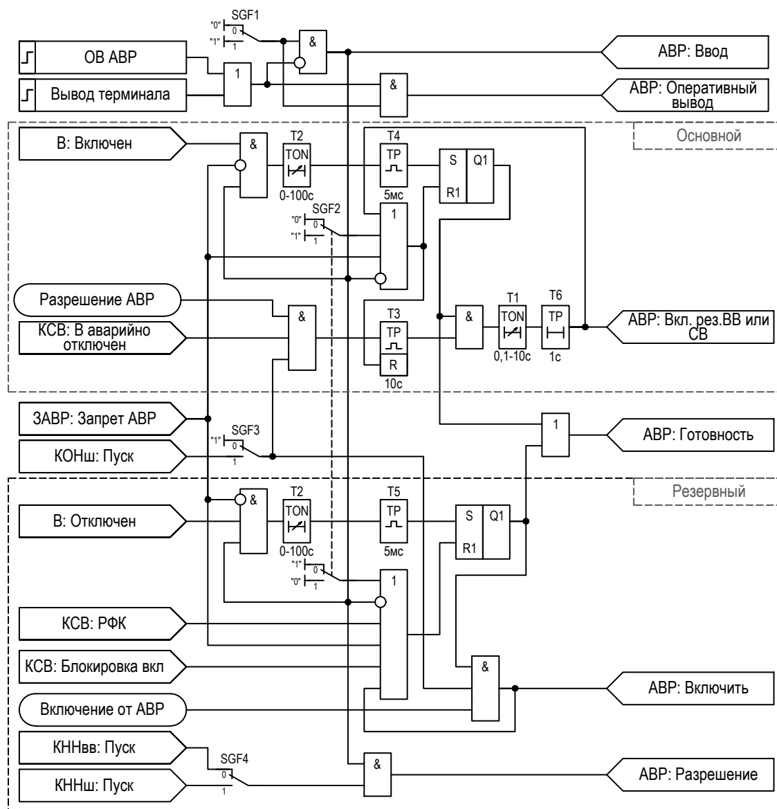
Рисунок 2.44 – Функциональная схема «ABP»
