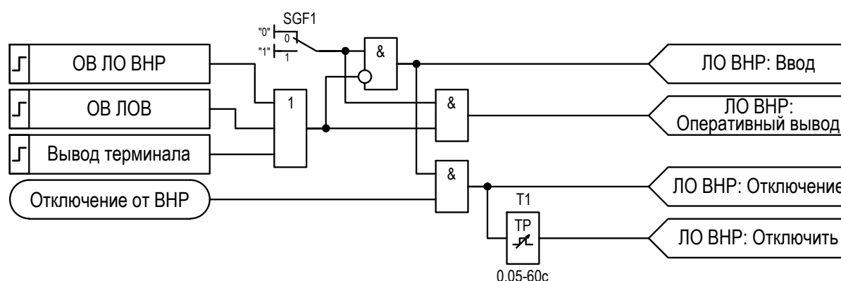
Рисунок 2.49 – Функциональная схема «ЛО ВНР»
