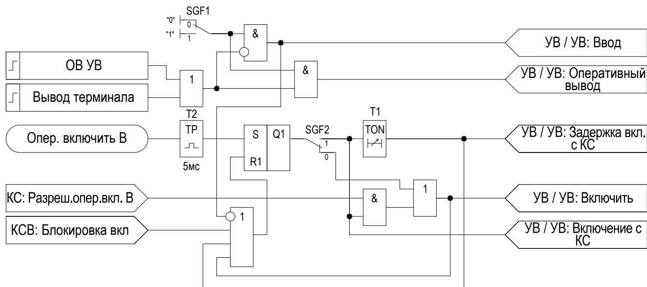
Рисунок 2.68 – Функциональная схема «УВ»
